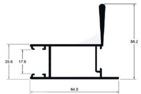
SU280 4,7 Kg PERFIL C/ 4,60
