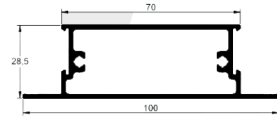
LG022 6,7 Kg | BR
