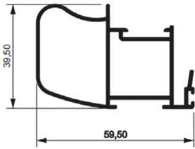
SU349 3,5 Kg PERFIL C/ 4,60
