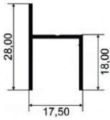
BX106 1,4 Kg - C/ 6 MT 1,0 kg - C/ 4 MT
