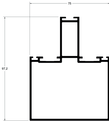
PAT202 11,8 Kg - C/ 6 MT 12,8 Kg - C/ 6,5 MT
