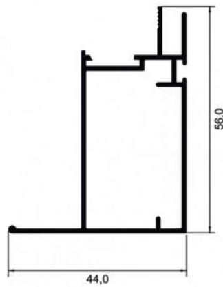
MP069 3,6 Kg PERFIL C/ 4,6
