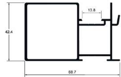
SU047 4,7 Kg PERFIL C/ 4,60
