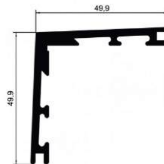
CL006 3,1 Kg 3,00 MT/BARRA
