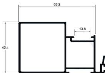
SU049 4,7 Kg PERFIL C/ 4,60
