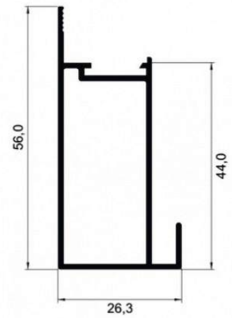
MP070 3 Kg PERFIL C/ 4,6
