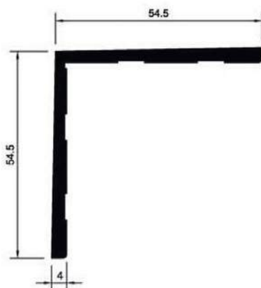
CL007 3 Kg 3,00 MT/BARRA
