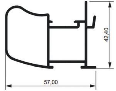
SU347 3,5 Kg PERFIL C/ 4,60
