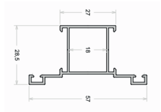
SU085 3,2 Kg | BR
