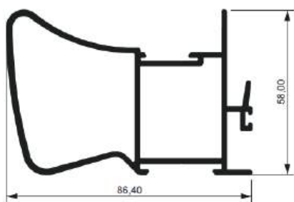
LG137 7,35 Kg - C/ 4,6 MT 9,0 Kg - C/ 6 MT
