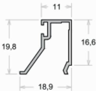
ALO27 1,05 Kg | BR
