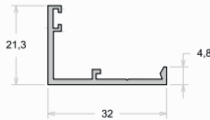
ALO26 1,4 Kg | BR
