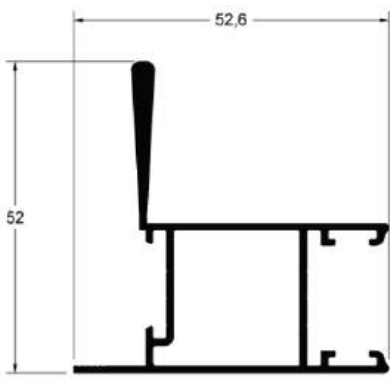
SU250 3,5 Kg PERFIL C/ 4,60
