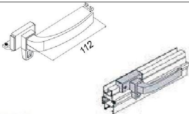
FEC-010 Fecho Direito p/ Maxi-ar s/ Baguete
